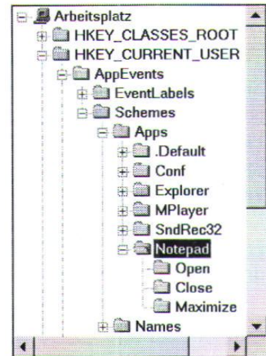
Abb 59: Einige neue Schlüssel machen Windows musikalisch
