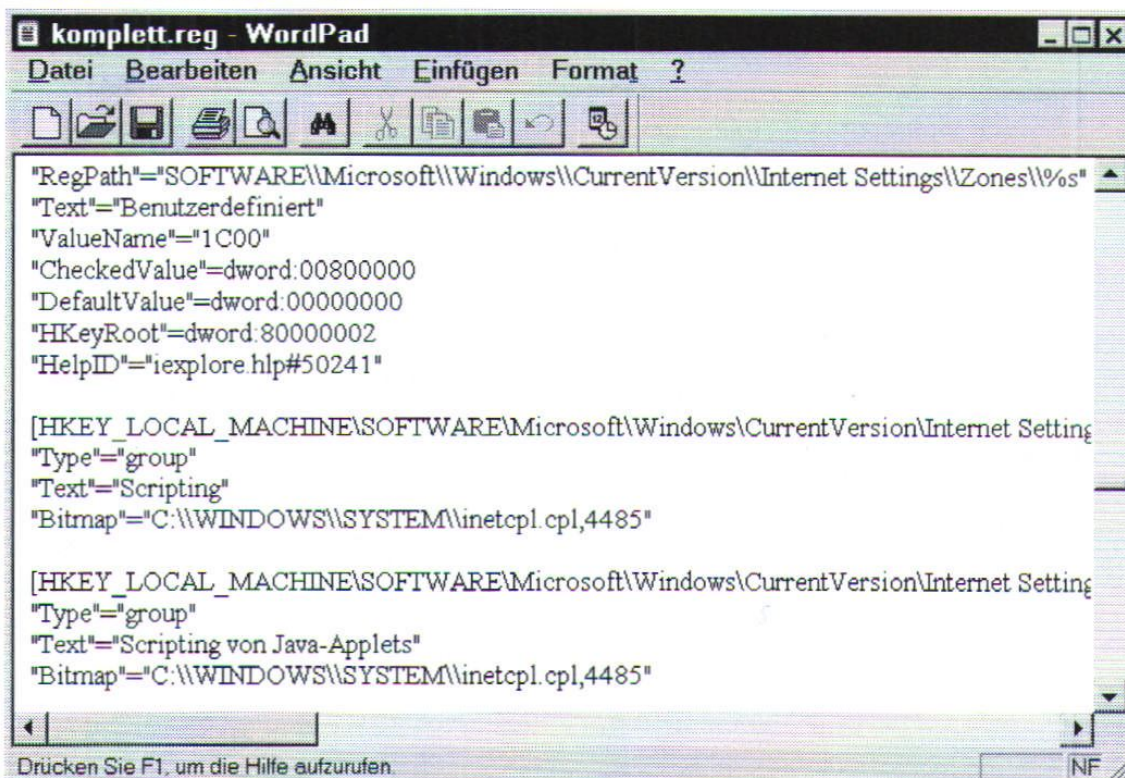
Abbildung 21: Die Registry in Textform als REG-Datei
