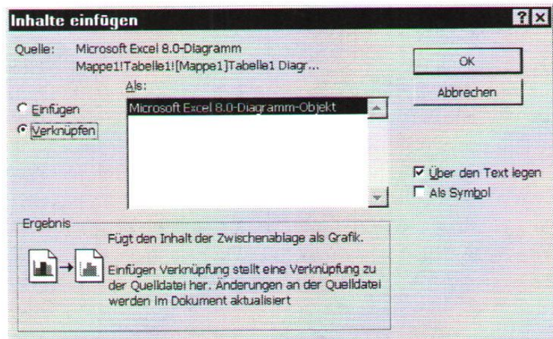
Abbildung 24: Verknüpfen bringt Aktualität
