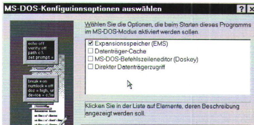
Abbildung 54: Hier fehlen einige wichtige Optionen
