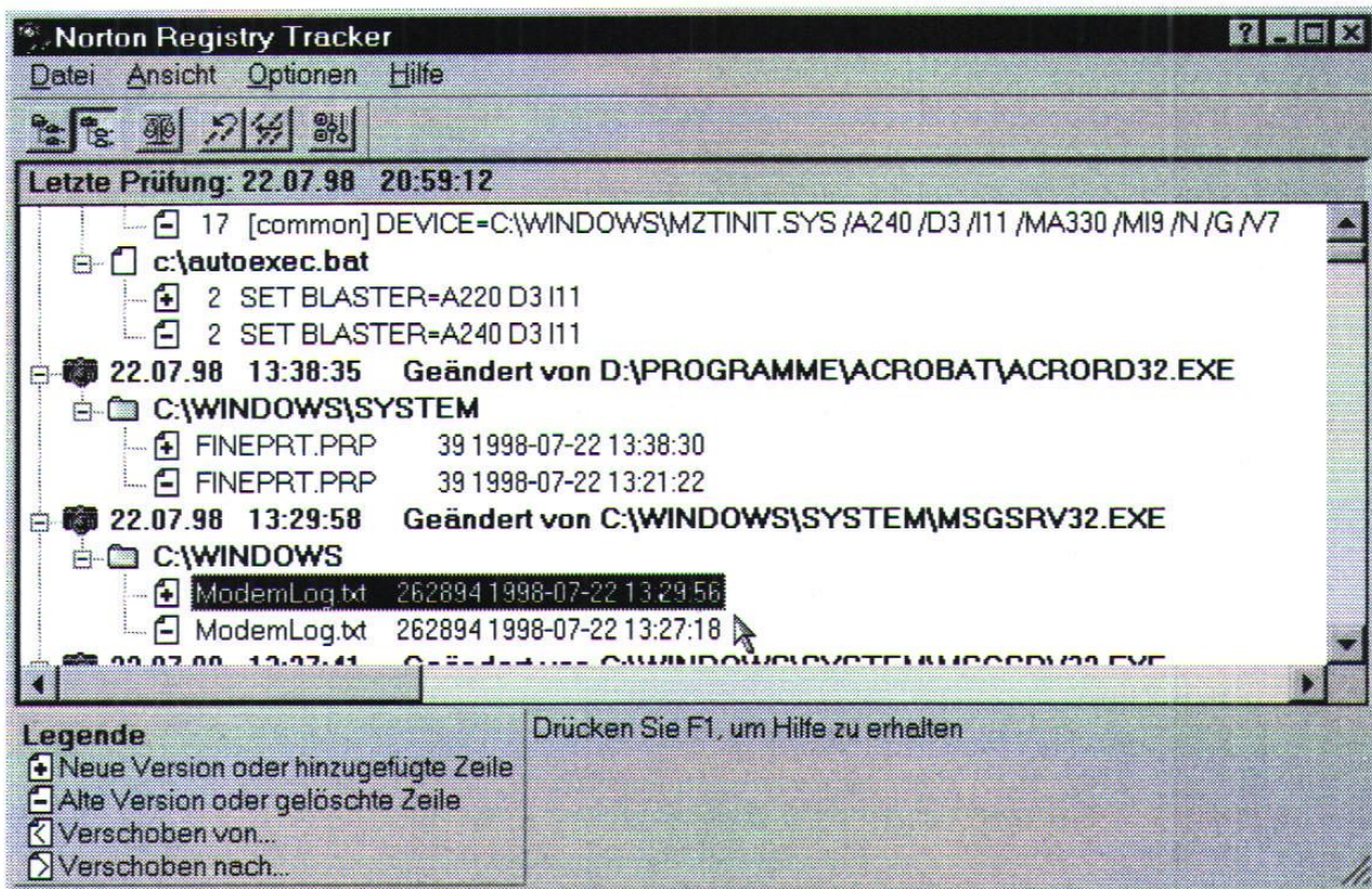
Abbildung 72: Der Registry-Tracker überwacht alle Änderungen
