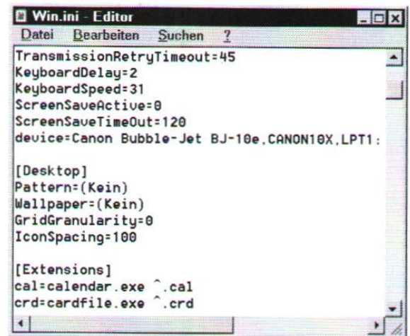
Abbildung 1: Eine klassische WIN.INI von Windows 3.1
