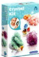
Kristalle züchten
